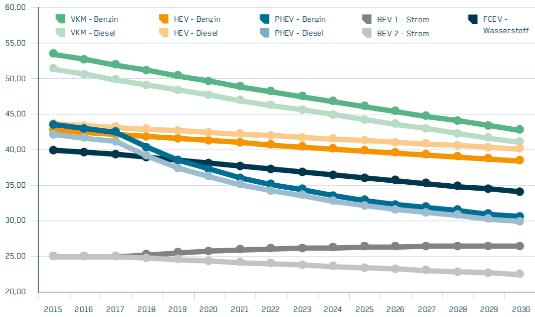
Abbildung 15: Abgeschätzte Entwicklung der Verbräuche der Neuzulassungen je Antriebsart in kWh/100km auf Basis der Durchschnittsverbräuche der Neuzulassungen von 2015 gem. PROVEM (s. Anhang S. 92)
