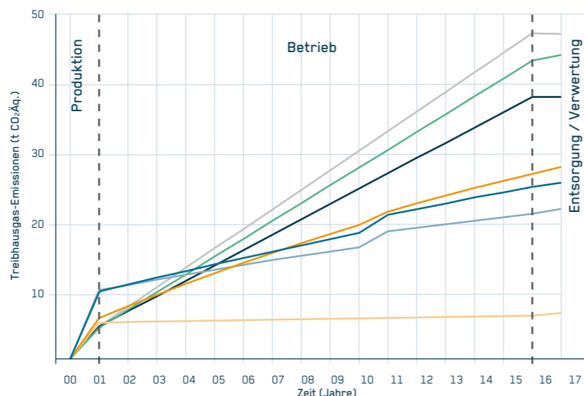
Abbildung 39: THG-Bilanz ausgewählter Antriebe im Lebenszyklus (IST-Szenario)
